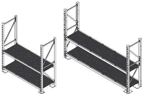
RK-2590 W.2550 D.900 H.2700 mm
