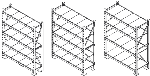
RK-2160 W.2150 D.600 H.2800 mm
