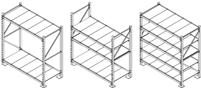
RK-2612-A W.2650 D.1200 H.2800 mm
